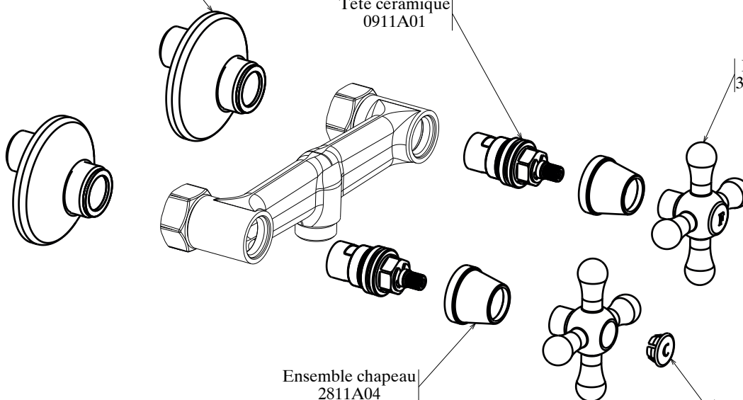
Ensemble rosace+excentrique 0898A00
